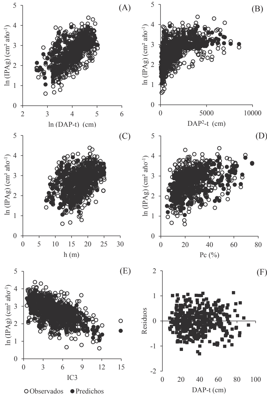
Figura 3. Valores observados y predichos de la ecuación de ajuste de incremento periódico en el área basal en función de cada variable independiente: A) \ln(DAP-t) : logaritmo del diámetro a la altura del pecho al inicio del periodo en centímetros; B) DAP^2-t : diámetro a la altura del pecho al cuadrado al inicio del periodo en centímetros; C) h : altura en metros; D) Pc\% : proporción de la copa; E) IC3 : índice de competencia; F) residuos en función del diámetro a la altura del pecho al inicio del periodo en centímetros.
